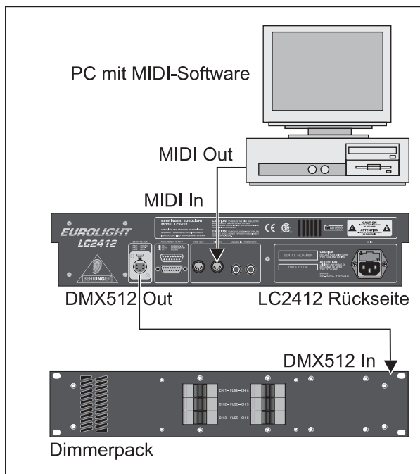
Abb. 7.4: MIDI-Verkabelung
